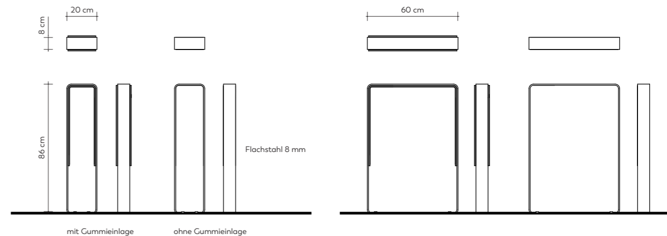
Fahrradständer groß
