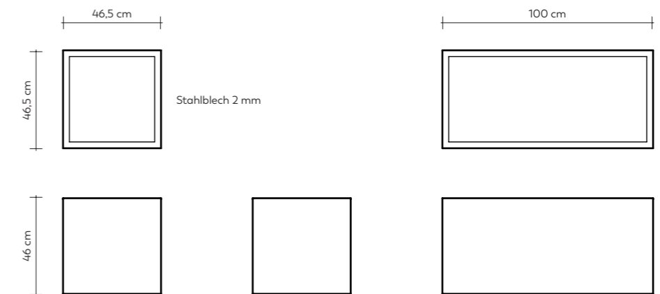
Pflanzkübel klein
