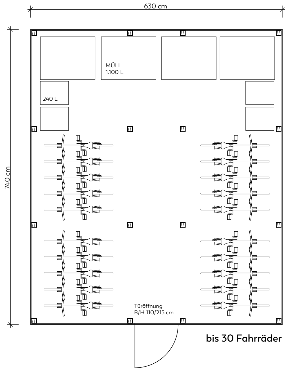
VARIOBOX 46 B 630 cm T 740 cm H 255 cm
