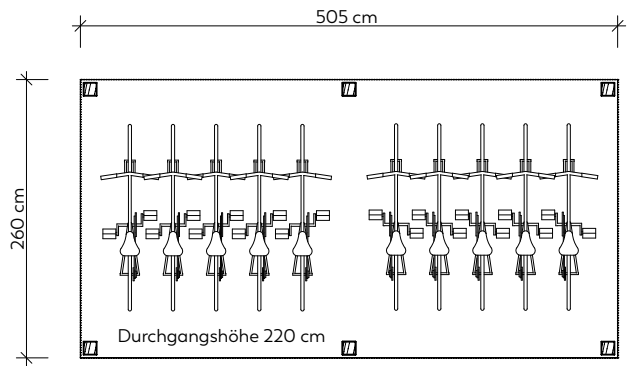
DACH 13 bis 10 Fahrräder
