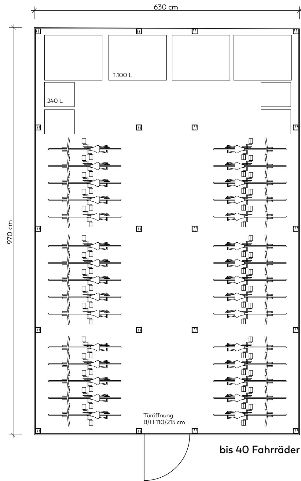
VARIOBOX 61 B 630 cm T 970 cm H 255 cm
